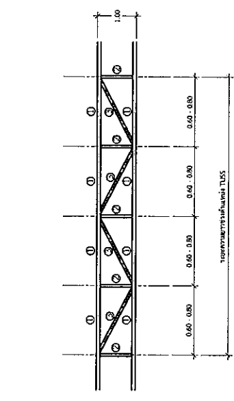
แปลนขยาย TUSS 1
