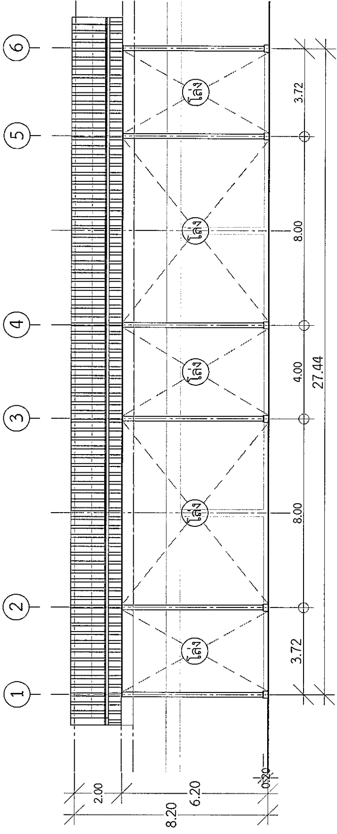
แปลนรูปด้าน B
