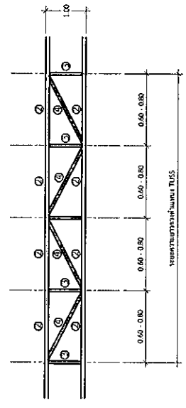
แปลนขยาย TUSS 2
